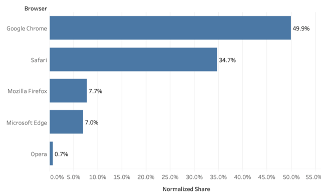
AI Metrics
