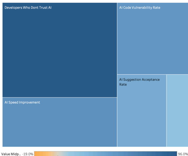
AI Metrics
